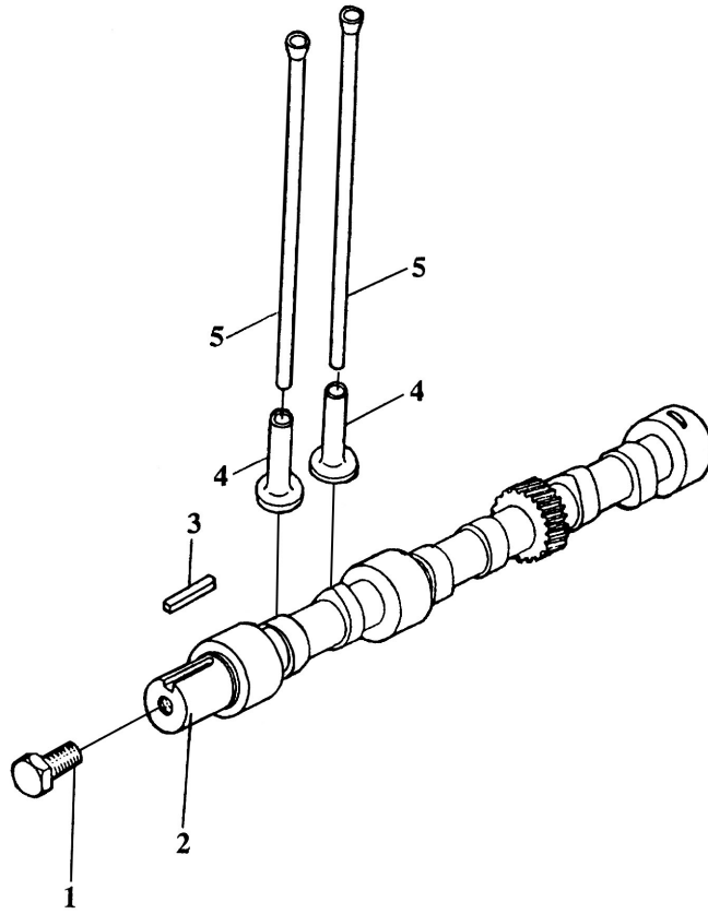
Fig. 6 Camshaft Assy(Y385)
